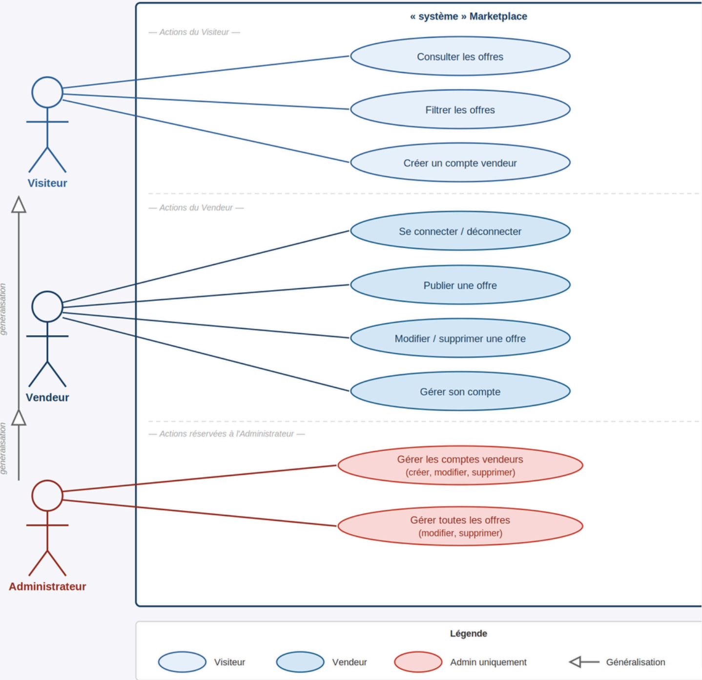
Diagramme de cas d'utilisation — Marketplace Particuliers
