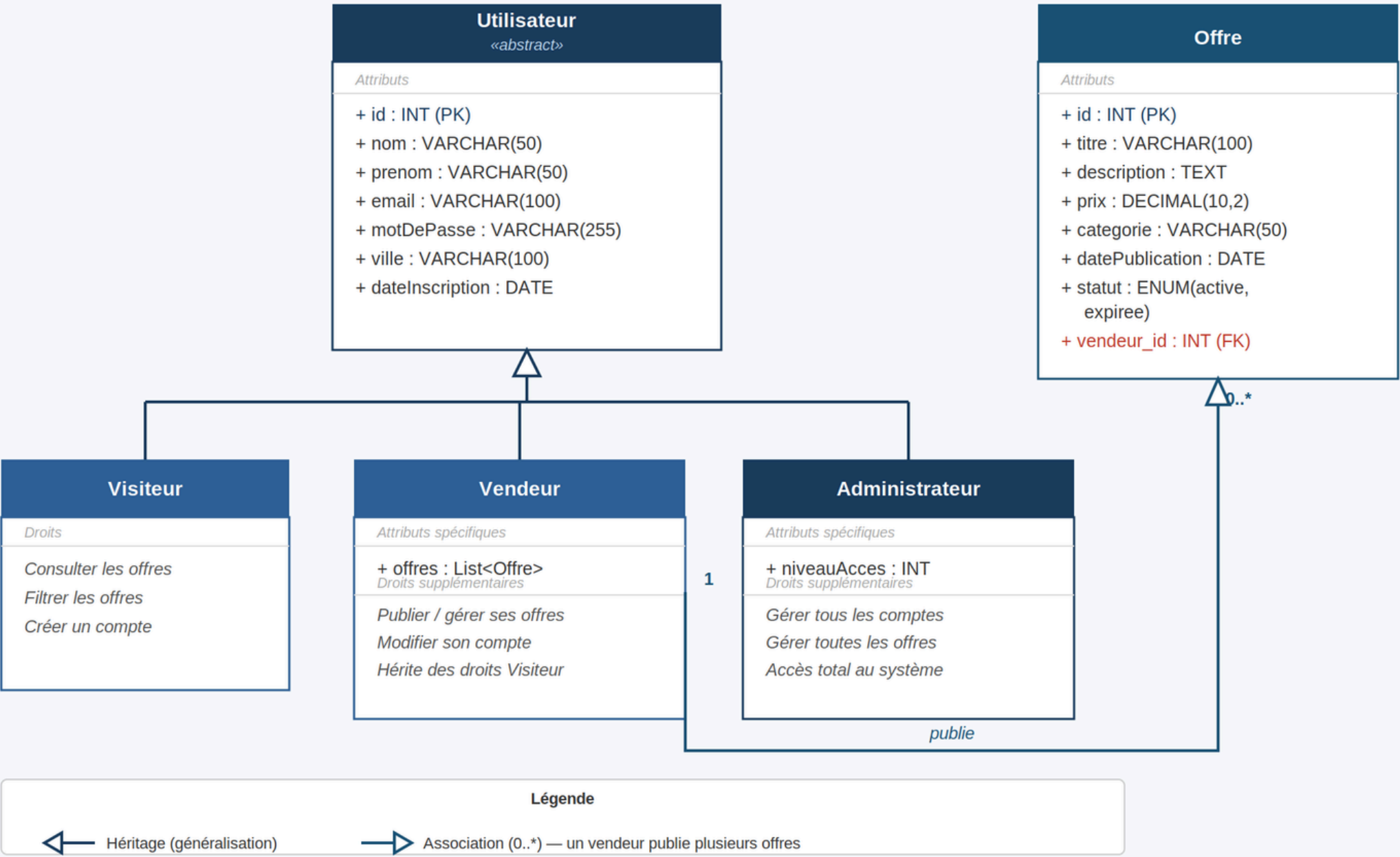
Diagramme de classes — Modèle de données
