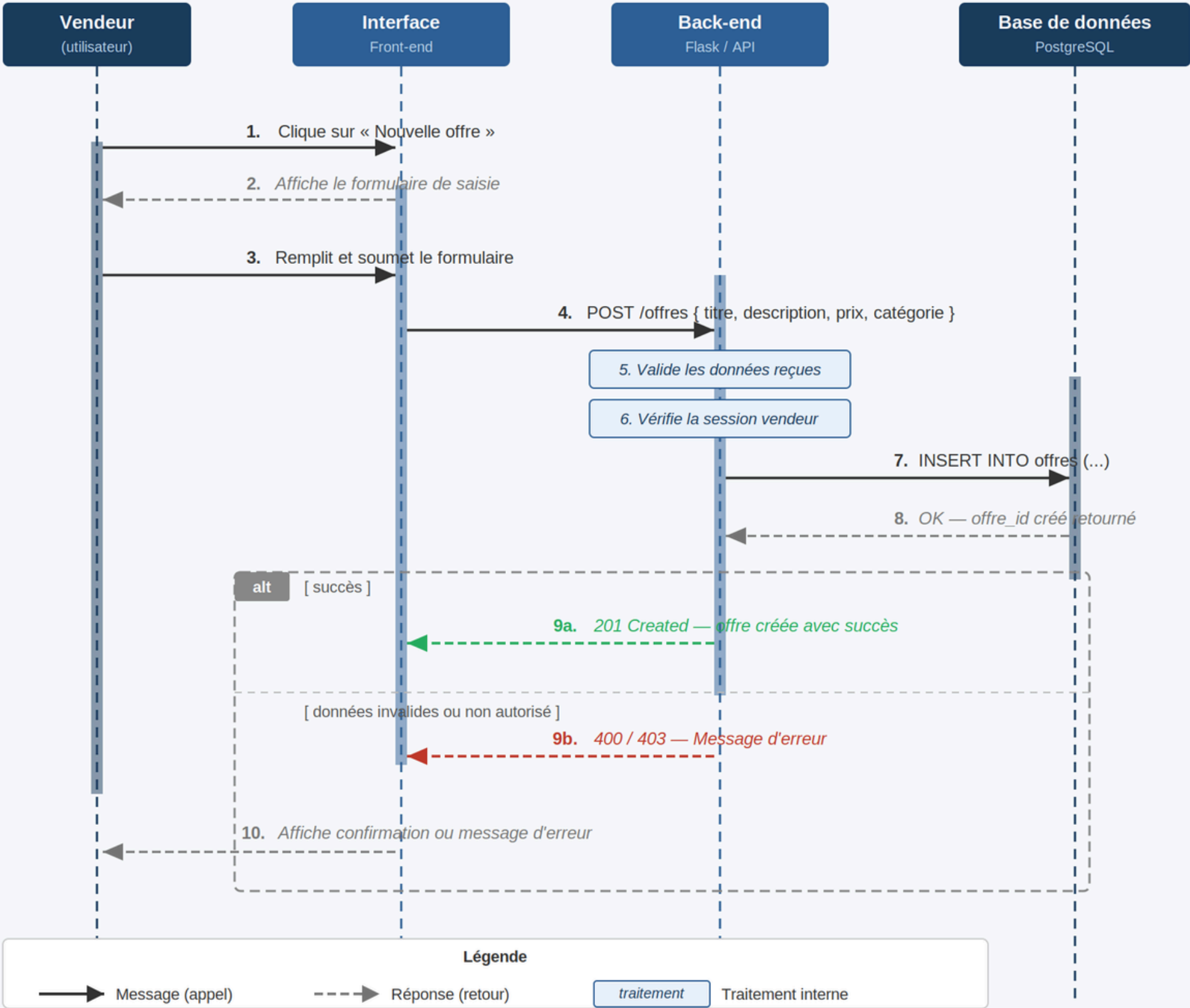
Diagramme de séquence — Création d'une offre par un vendeur
